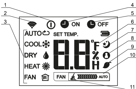
Рисунок 4 - индикационный дисплей пульта дистанционного управления
